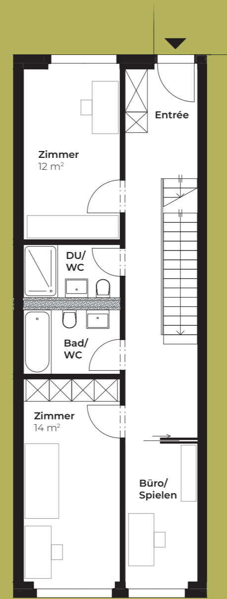
OBERGESCHOSS
